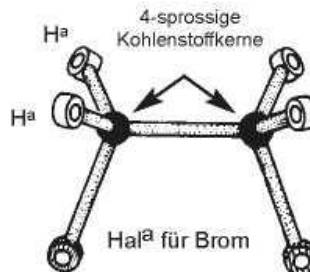
Abbildung 2 Dibromethan
