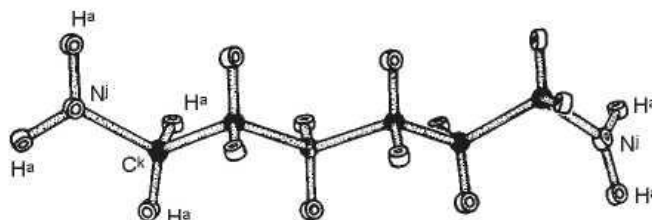
Abbildung 1 \text{H}_2\text{N}\cdot\text{CH}_2\cdot\text{CH}_2\cdot\text{CH}_2\cdot\text{CH}_2\cdot\text{CH}_2\cdot\text{NH}_2
