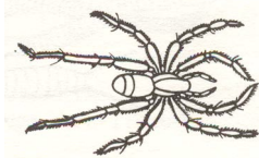
Wolfsspinne (2 cm)
