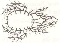
Ohrwurm (2 cm)
