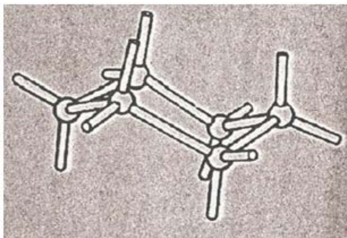
Model cykloheksanu
